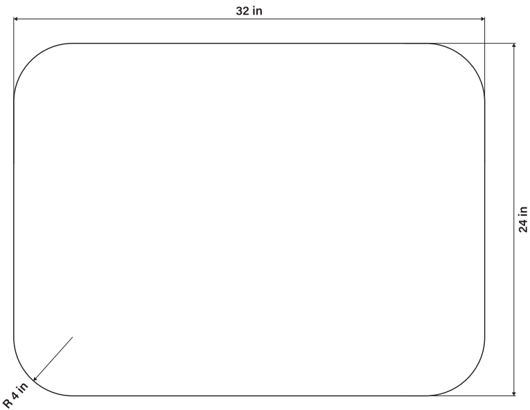
OBJECT 005 - TOP
