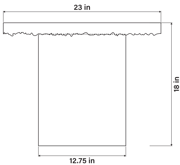
OBJECT 011 SIDE TABLE - SIDE
